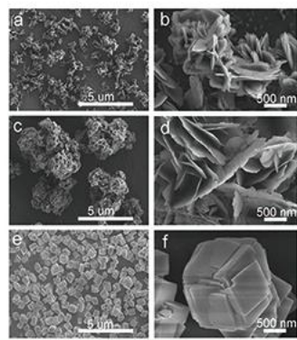
李守柱教授课题组研发MOF材料的扫描电镜
